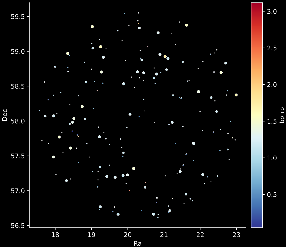
APOGEE DR17 Field: [CVZTILE_088+24_btx] Stars: 185
