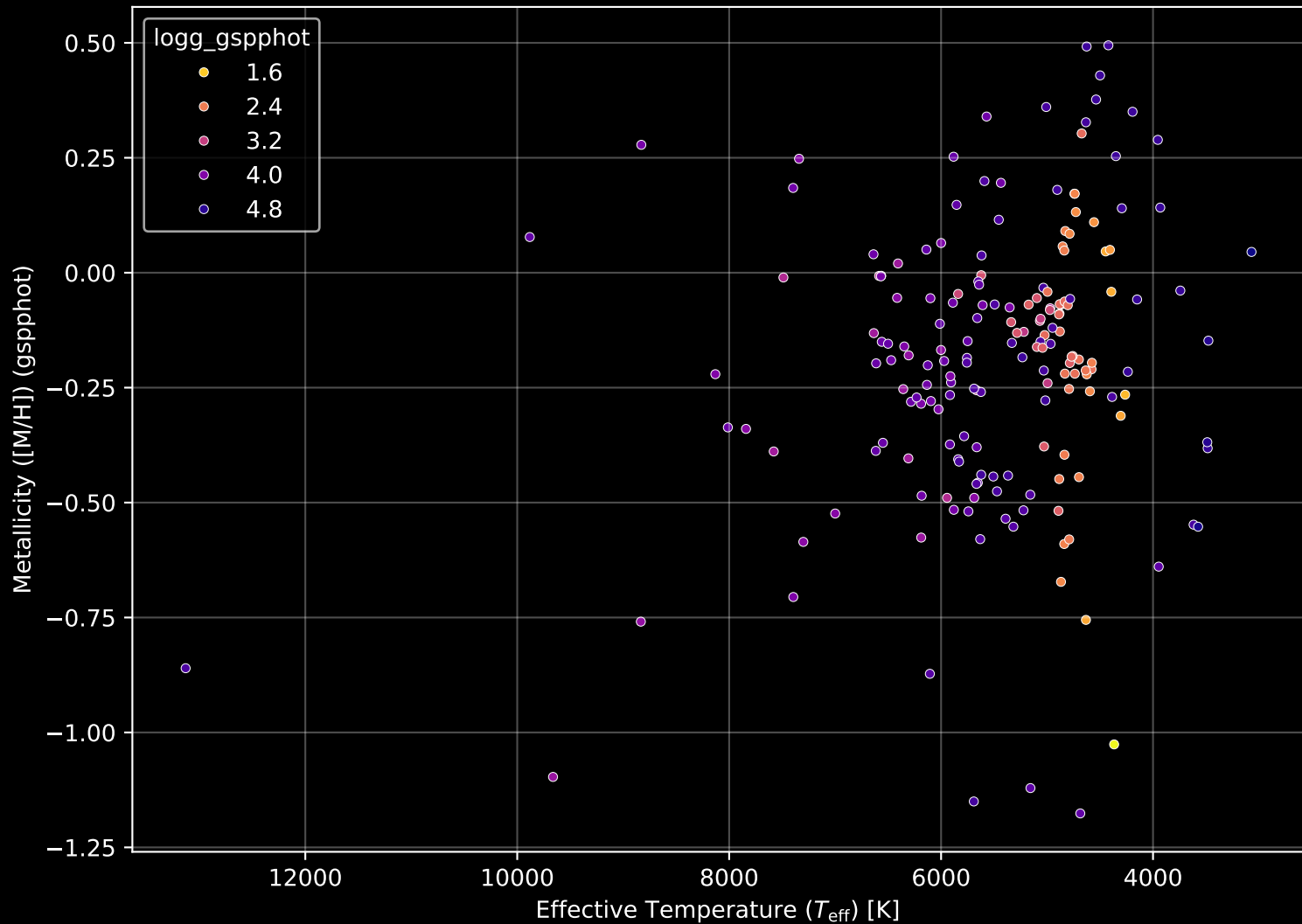
APOGEE DR17 Field: [CVZTILE_088+24_btx] Stellar Population Parameters (n= 185)
